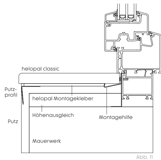
bündiger Einbau bei Ziegel-Massiv
