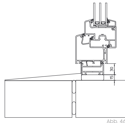
Montage während der Fassadenarbeiten - Fensterbank eingeputzt
