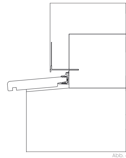
Beispiel: Leitdetail einer Nutausbildung
