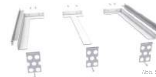
Einbau mit Montageset - passend für Schattennutprofil 4 und 5 mm (Erweiterungsset für Fensterbänke ab 1,50 m erhältlich)
