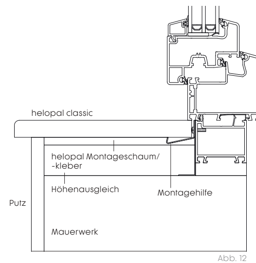
klassischer Einbau bei Ziegel-Massiv
