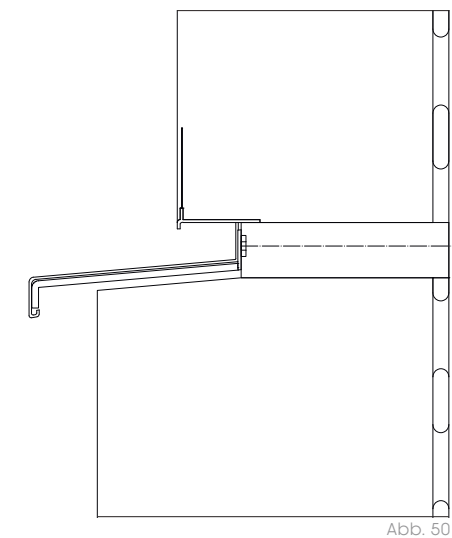
Beispiel: Leitdetail einer Nutausbildung
