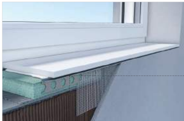
Einbau bei Ziegelparapet mit verputzter Fläche
