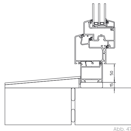
Nachträgliche Montage - Fensterbank nicht eingeputzt. Zweite wasserführende Ebene erforderlich.
