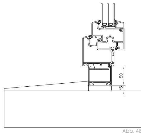
Monolithisches Mauerwerk
