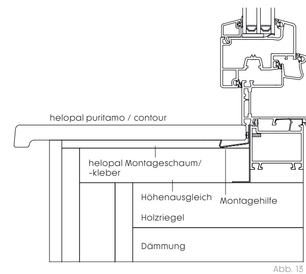
klassischer Einbau im Holzriegel
